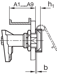
门锁 GN 119
