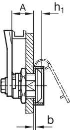
门锁 GN 115
